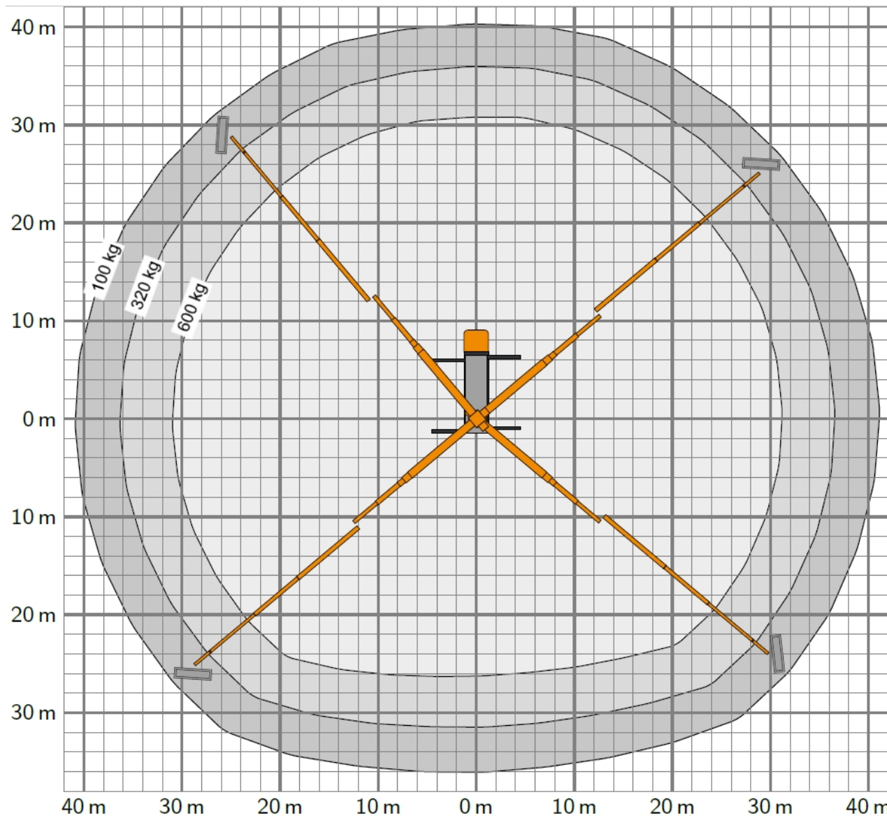
WERKDIAGRAM RUTHMANN T700HF / T720 - BOVENAANZICHT
